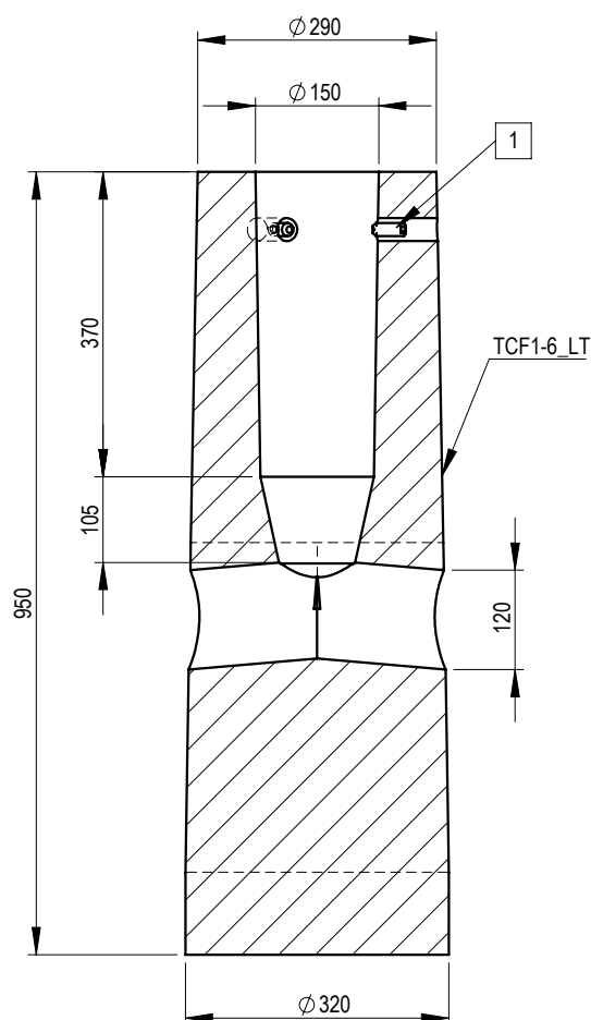
SEC. A-A (1 : 10)
